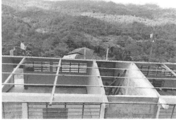
Foto 1: Área de la parte de atrás donde se está realizando el mejoramiento de tubos galvanizados para la cubierta de lámina.
